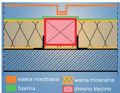
Przekrój izolacji akustycznej kopuły
